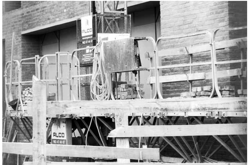
Aquesta plataforma elevadora no compta amb una barana cega que eviti la caiguda dels maons apilats
