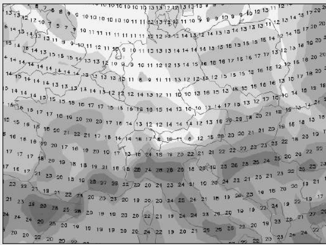
Temperatures en superfície el 26 de maig a les 12 del migdia
