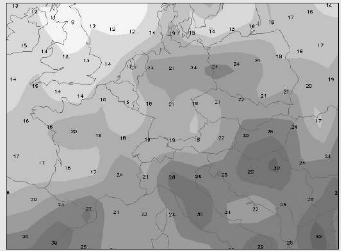
Temperatures en superfície el 8 de juny a les 12 del migdia
