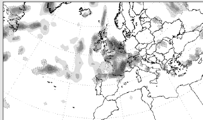
Precipitacions a les 18h del dimarts 4 de juliol. Tempestes al nord de Catalunya.
