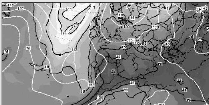
Temperatures dissabte 1 de juliol a les 18h a 1500 metres d'altura. Bombolla càlida.
