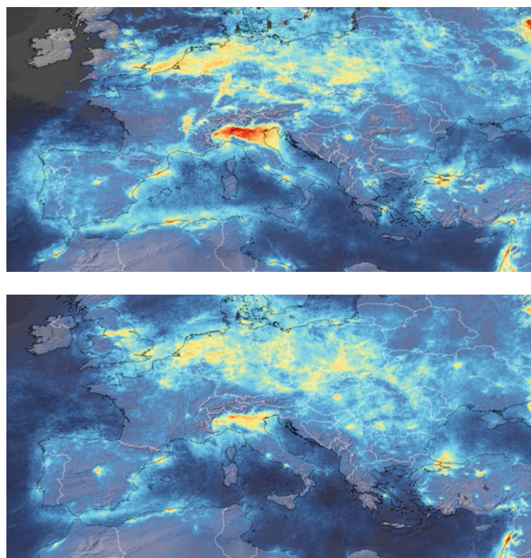
Concentració de diòxid de nitrogen ( \text{NO}_2 ) el gener i el març de 2020
