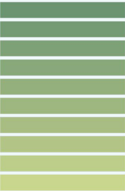
Les reserves de carboni a les praderies mortes són deu vegades superiors a les presents al sòl forestal
